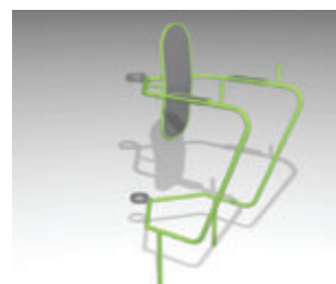
Навіс для преса в зборі OF-E.4
